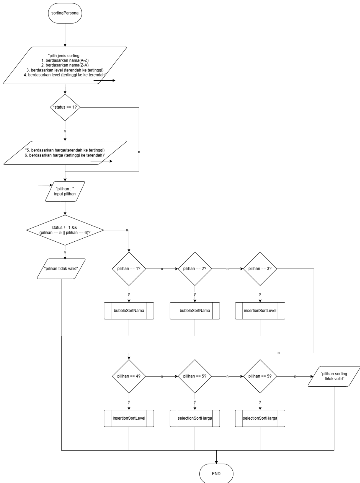
gambar 1.10 opsi user dan admin (menu sorting data persona)
