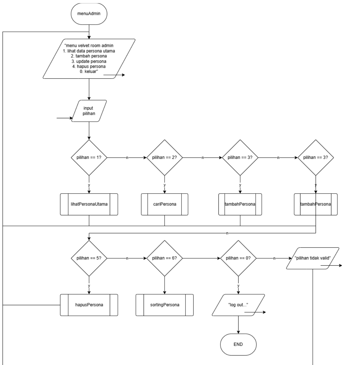
gambar 1.4 flowchart fungsi menuAdmin
