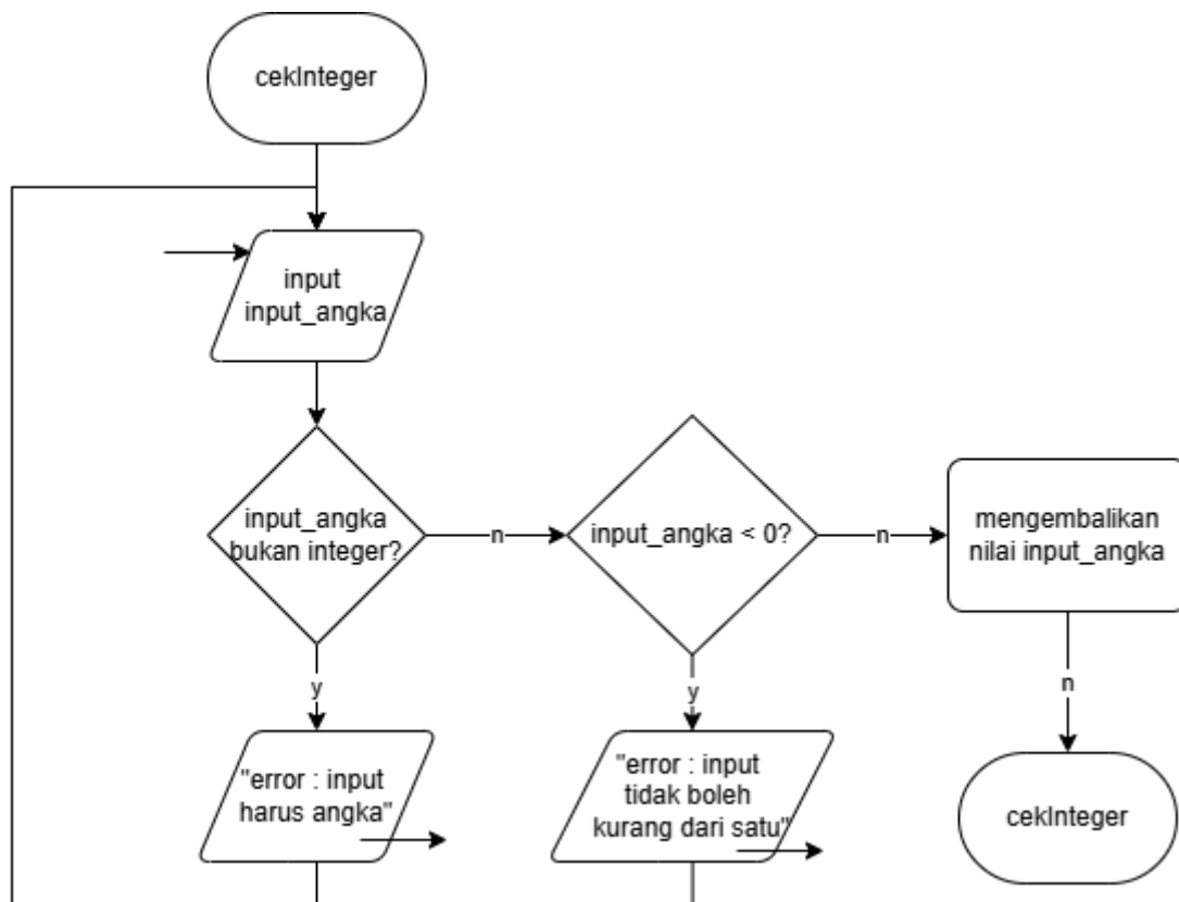
1.15 error handling input integer
