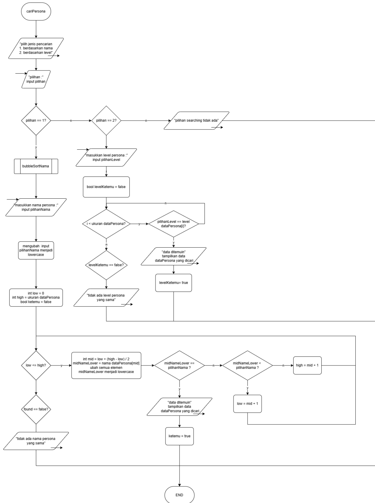
1.14 fungsi user dan admin (cari persona)
