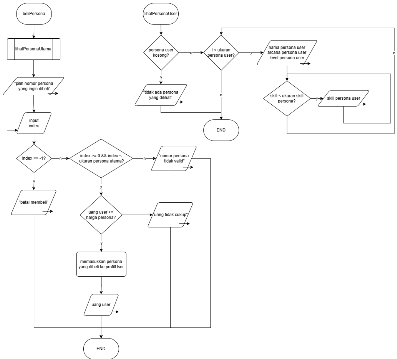
gambar 1.5 flowchart opsi user (fungsi beli dan lihat persona)
